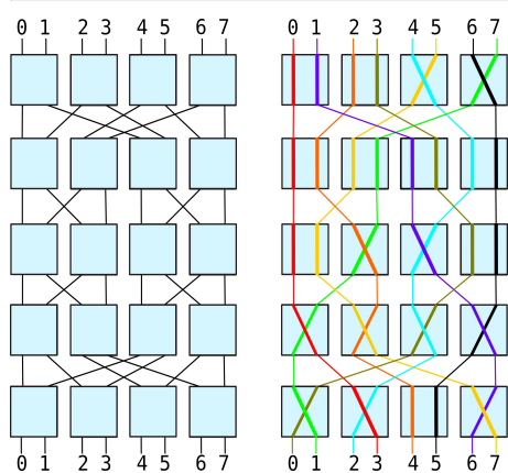
3-Beneš network
